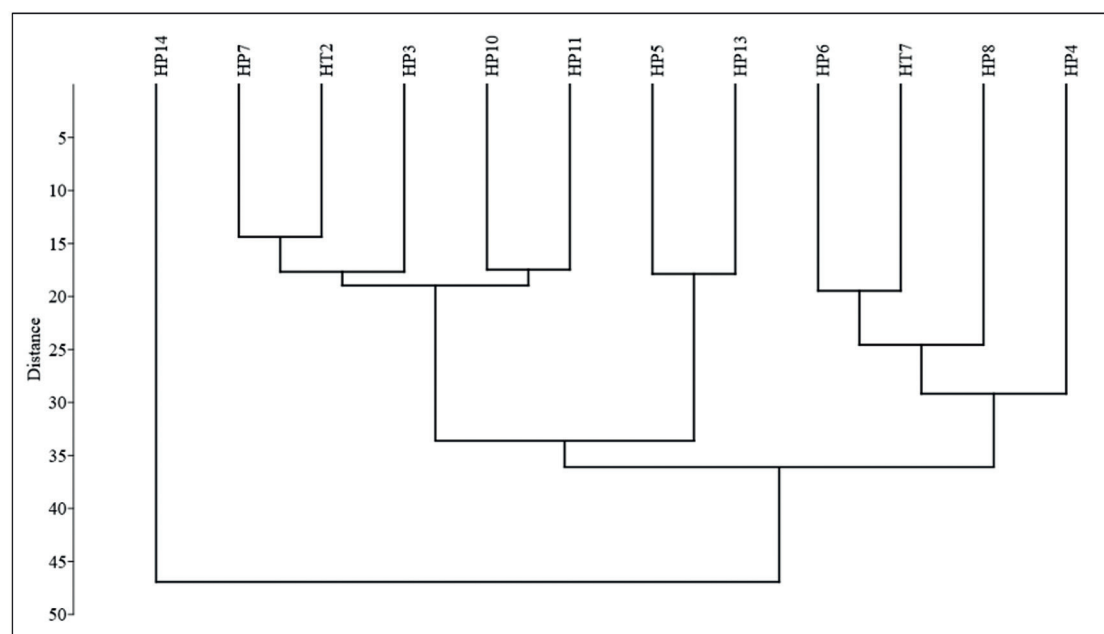
FIGURA 3: Dendrograma de 17 variables de plantas y frutos de huertas seleccionadas, con cuatro grupos definidos y tres sin definir a distancia euclidiana de 20.
